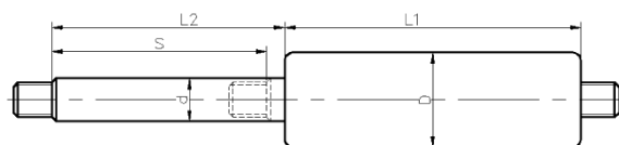
L1-缸筒长度 L2-活塞杆伸出长度 D-缸筒直径 d-活塞杆直径 S-行程
